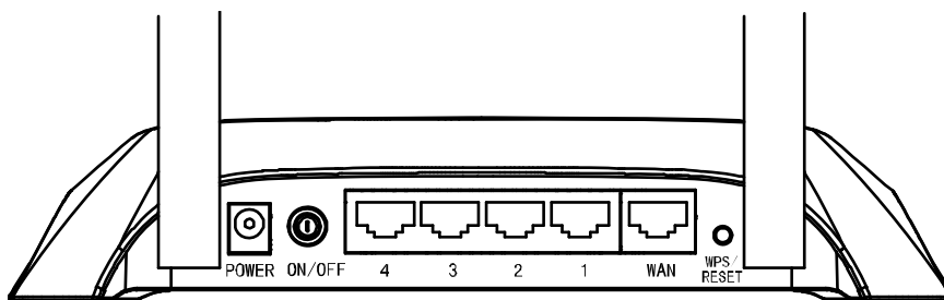
Рис. 1-2 Задняя панель
