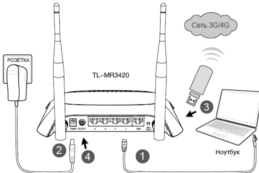
Рис. 2-1 Установка аппаратной части маршрутизатора TL-MR3420 - Сеть 3G/4G
