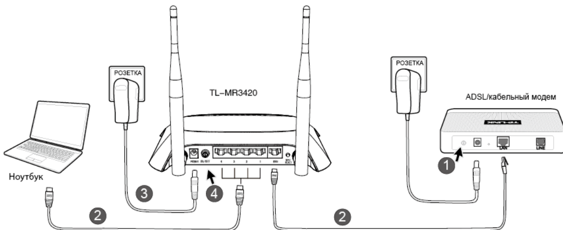
Рис. 2-2 Установка аппаратной части маршрутизатора TL-MR3420 - Сеть WAN
